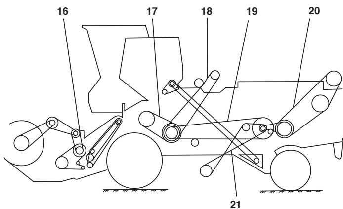
С КОПНИТЕЛЕМ
