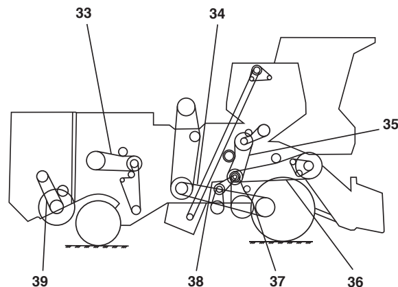
С МЕХ. ПРИВ. ХОДОВ. ЧАСТИ И ИЗМЕЛЬЧИТЕЛЕМ
