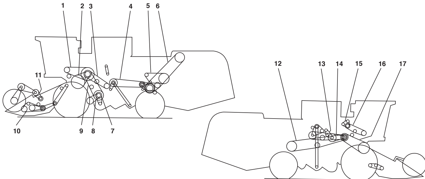
ИЗМЕЛЬЧИТЕЛЬ ПКН1500
