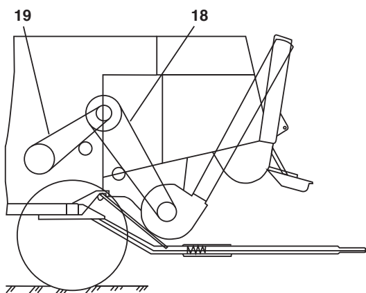
ИЗМЕЛЬЧИТЕЛЬ ПКН1500
