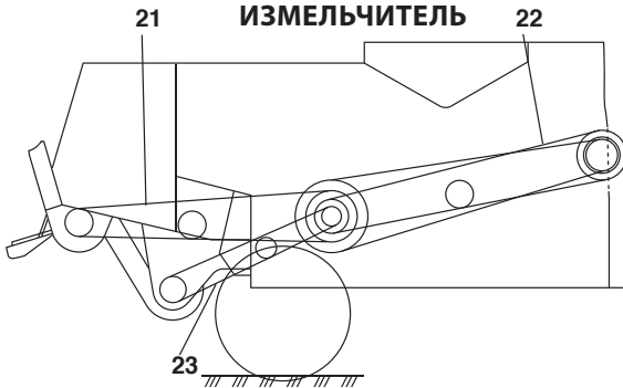
ИЗМЕЛЬЧИТЕЛЬ
