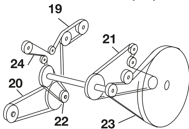
TX 62-64-65-66 (RH)
