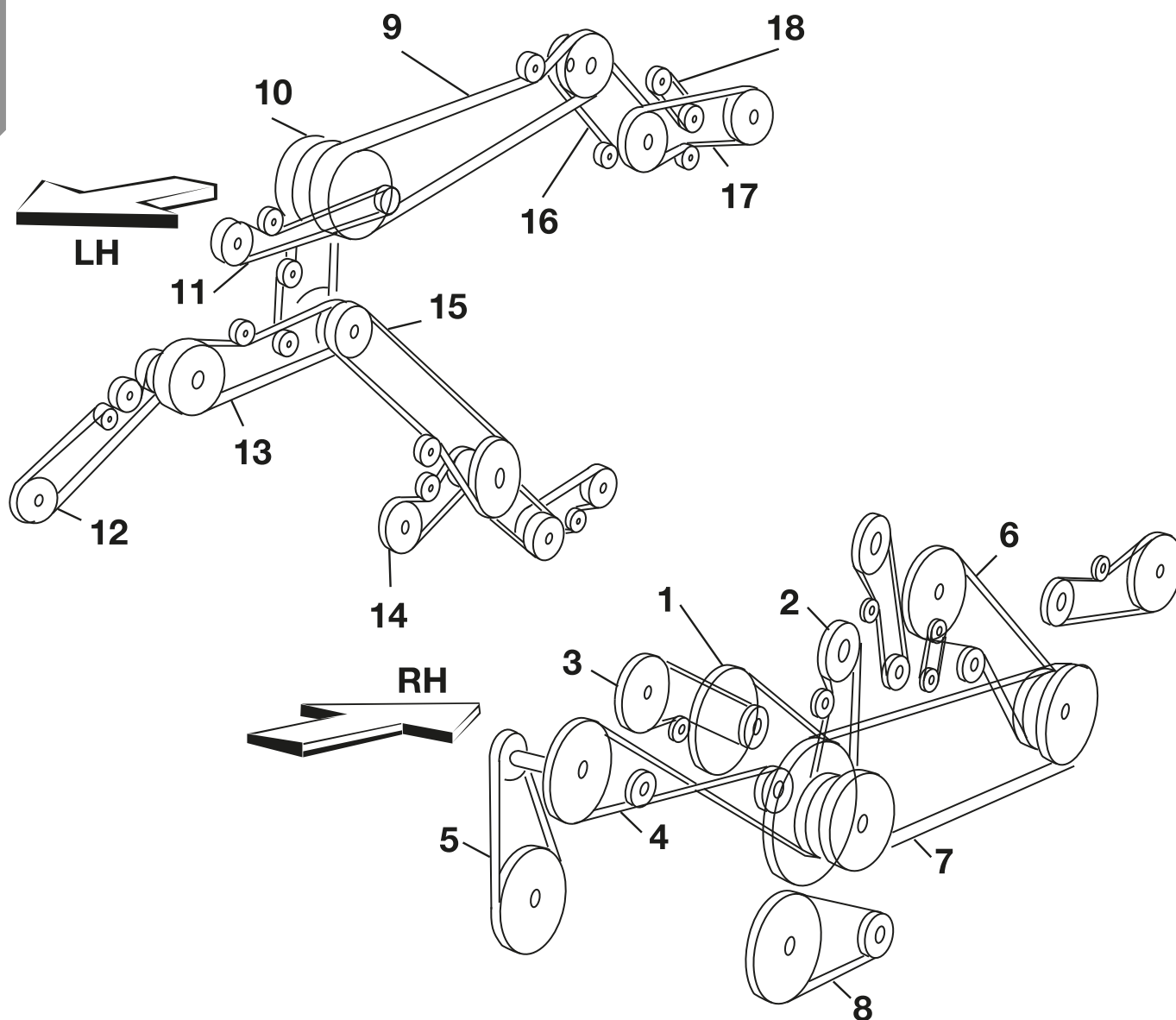
TX 62-64-65-66 (RH)
